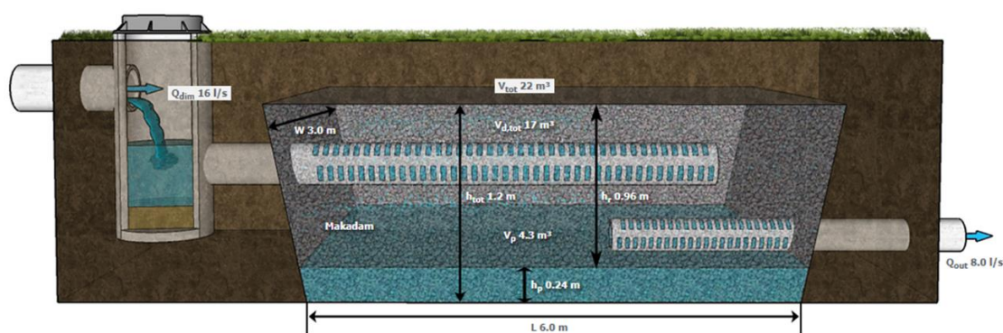
Figur 18. Skiss över ett makadammagasin (Bild: StormTac)
