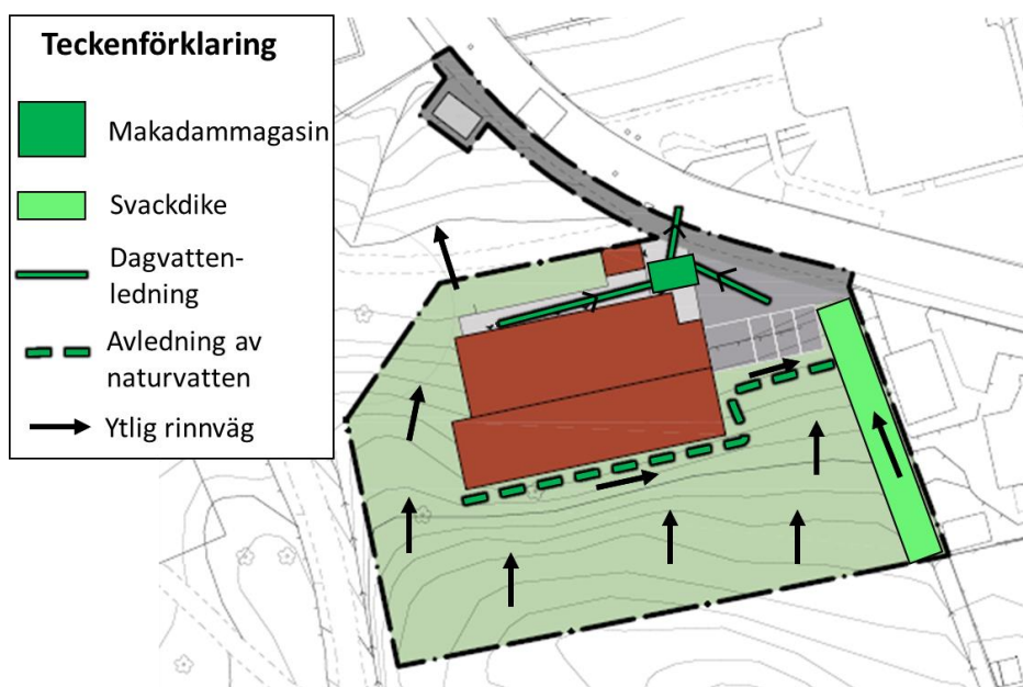
Figur 1. Föreslagen dagvatten- och skyfallshantering inom planområdet
