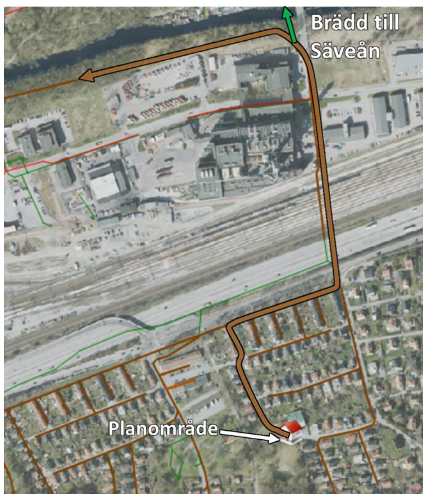
Figur 10. Kombinerat ledningssystem nedströms planområdet. Närmast nedströms bräddpunkt till Sävån visas i figur.
